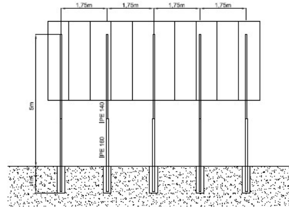
ALÇAT POSTERIOR Esc: 1/8
