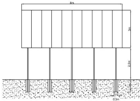
ALÇAT FRONTAL Esc: 1/8
